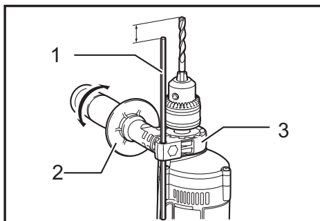
► 1. Calibrador de profundidad 2. Empuñadura lateral 3. Base de la empuñadura
